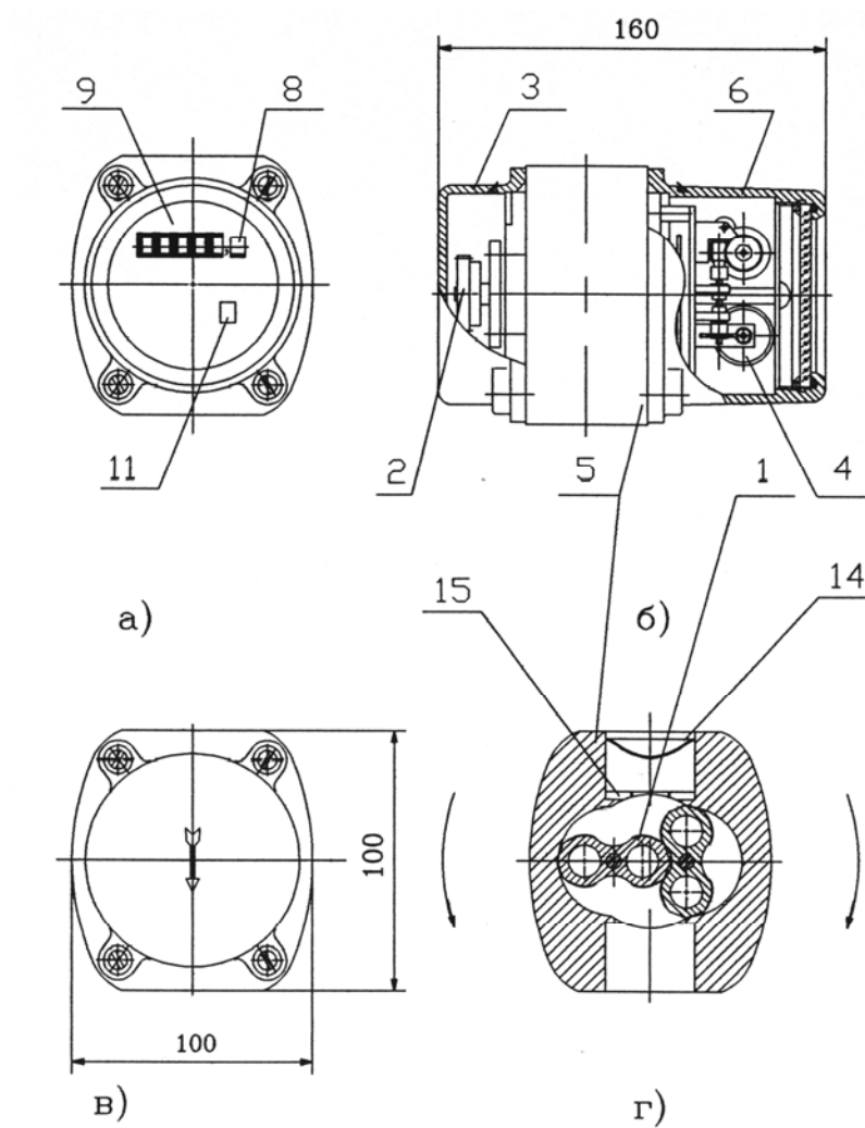
а) вид спереди; б) счетчик в разрезе; в) вид сзади г) устройство измерительной камеры
